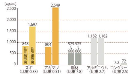
各素材の比圧縮・比引張強度
